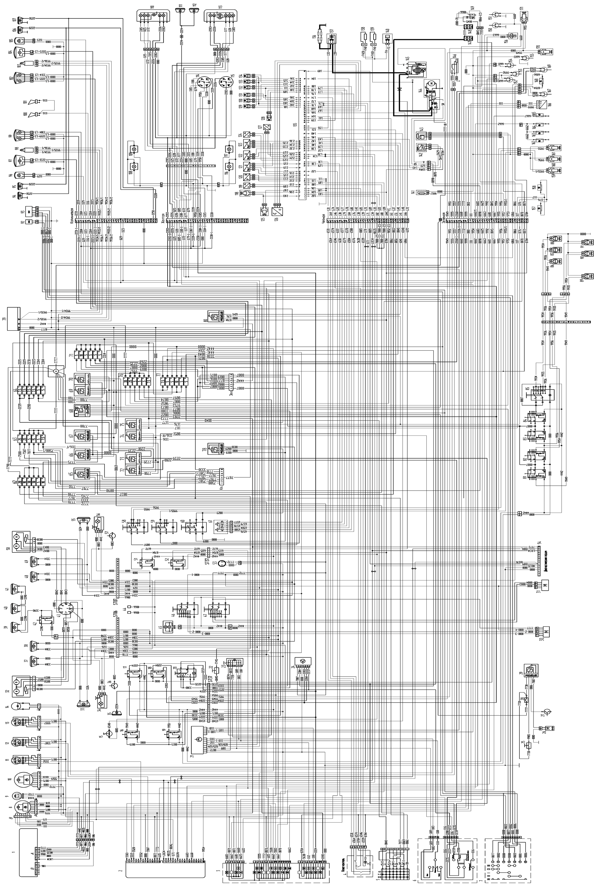
Рисунок Е.1- Схема электрооборудования автомобиля Урал-6370
